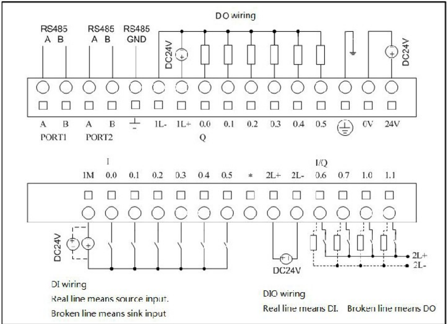
Рис. 2-1 Схема подключения K205-16DT
